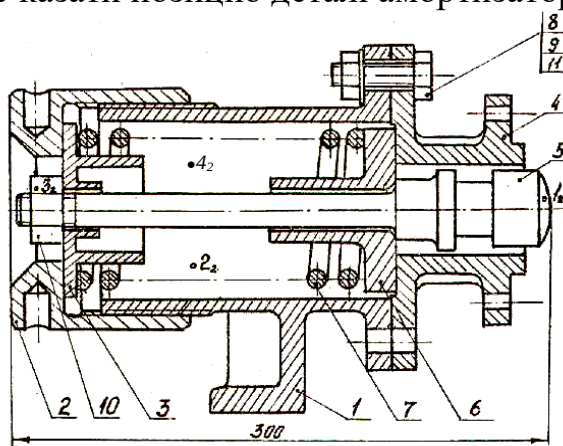
АМОРТИЗАТОР
